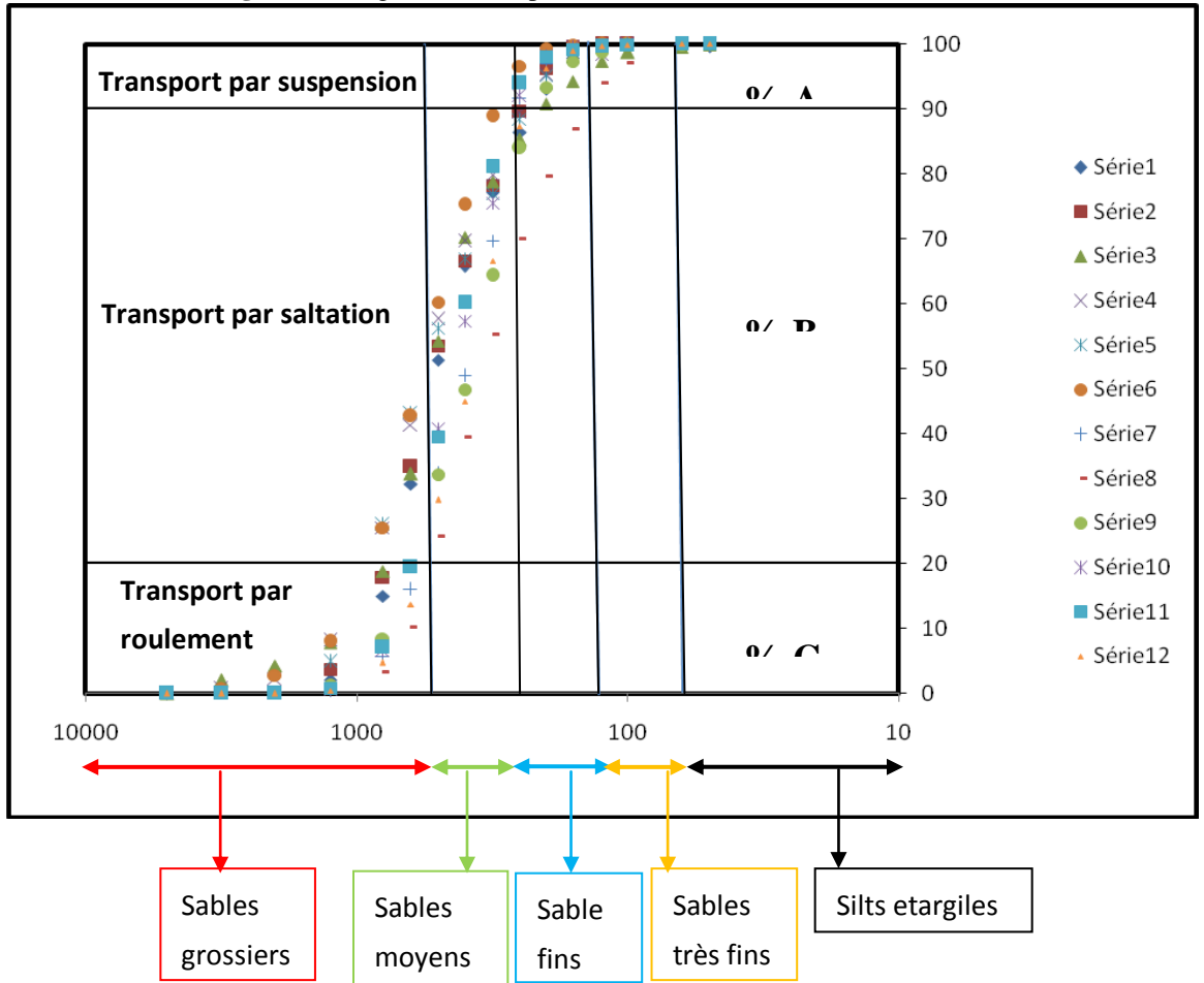
Figure 6 : Diagramme de répartition des sables selon le test de Visher
